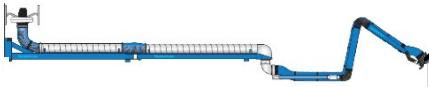
301 ΕΡΓΟΣΤΑΣΙΟ ΒΑΣΕΩΣ ΒΡΑΧΙΟΝΑΣ NEDERMAN HD ΣΕ ΠΡΟΕΚΤΑΣΗ 6,0m
