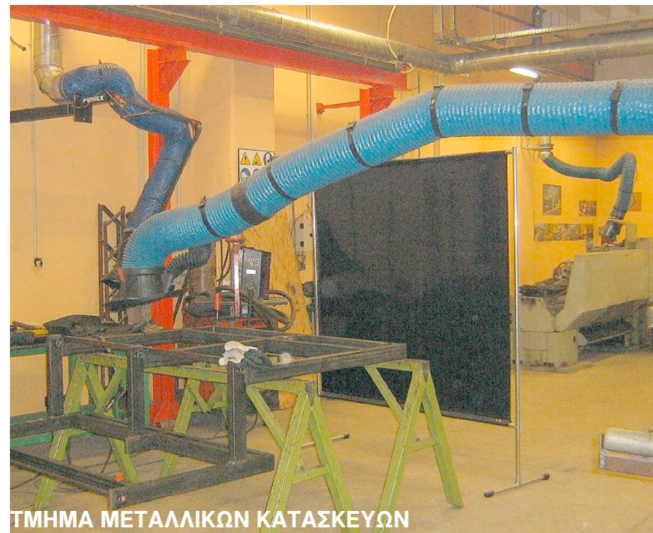
ΦΙΛΤΡΟ ΣΚΟΝΗΣ ΚΑΙ ΑΝΑΘΥΜΙΑΣΕΩΝ-ΤΜΗΜΑ ΜΕΤΑΛΛΙΚΩΝ ΚΑΤΑΣΚΕΥΩΝ
